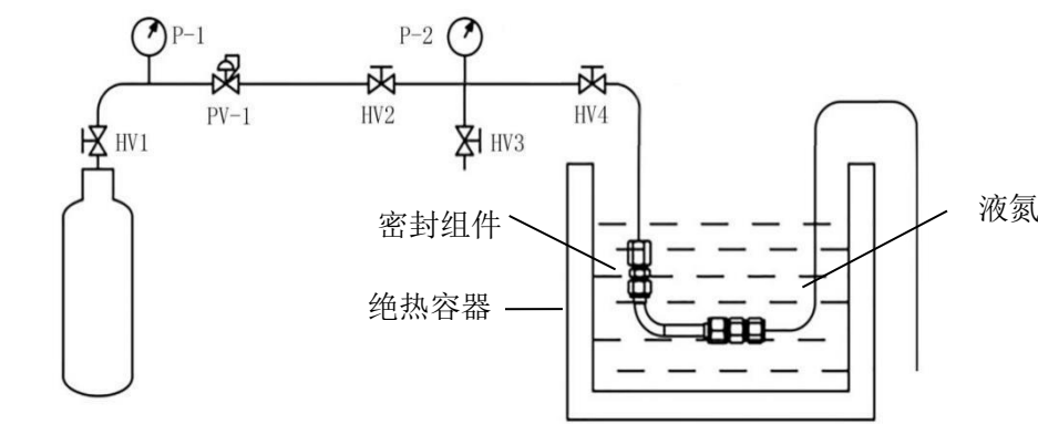
图3 低温气密性试验布置示意图
