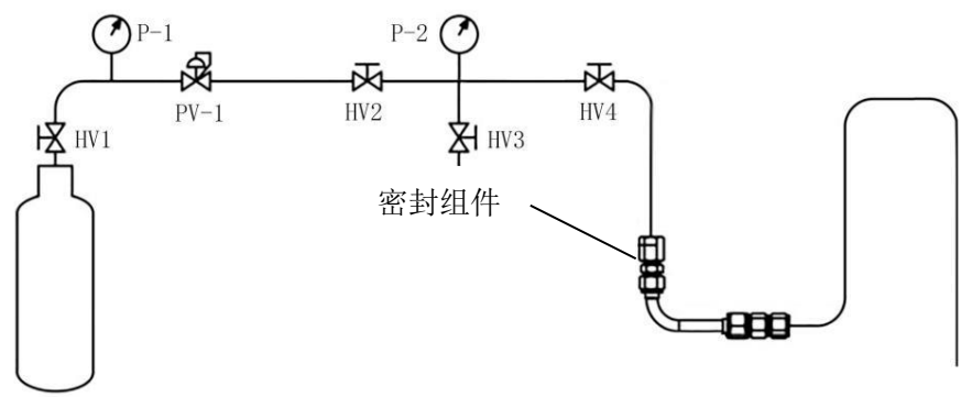
图2 常温气密性试验布置示意图
